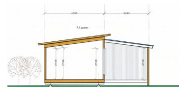
SNITT
